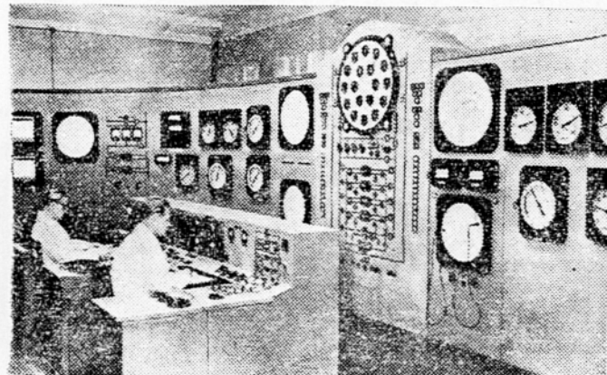
Agencije so te dni objavile prvo sliko kontrolne mize in naprav atomski električni centrali špajltske akademije znanosti.
