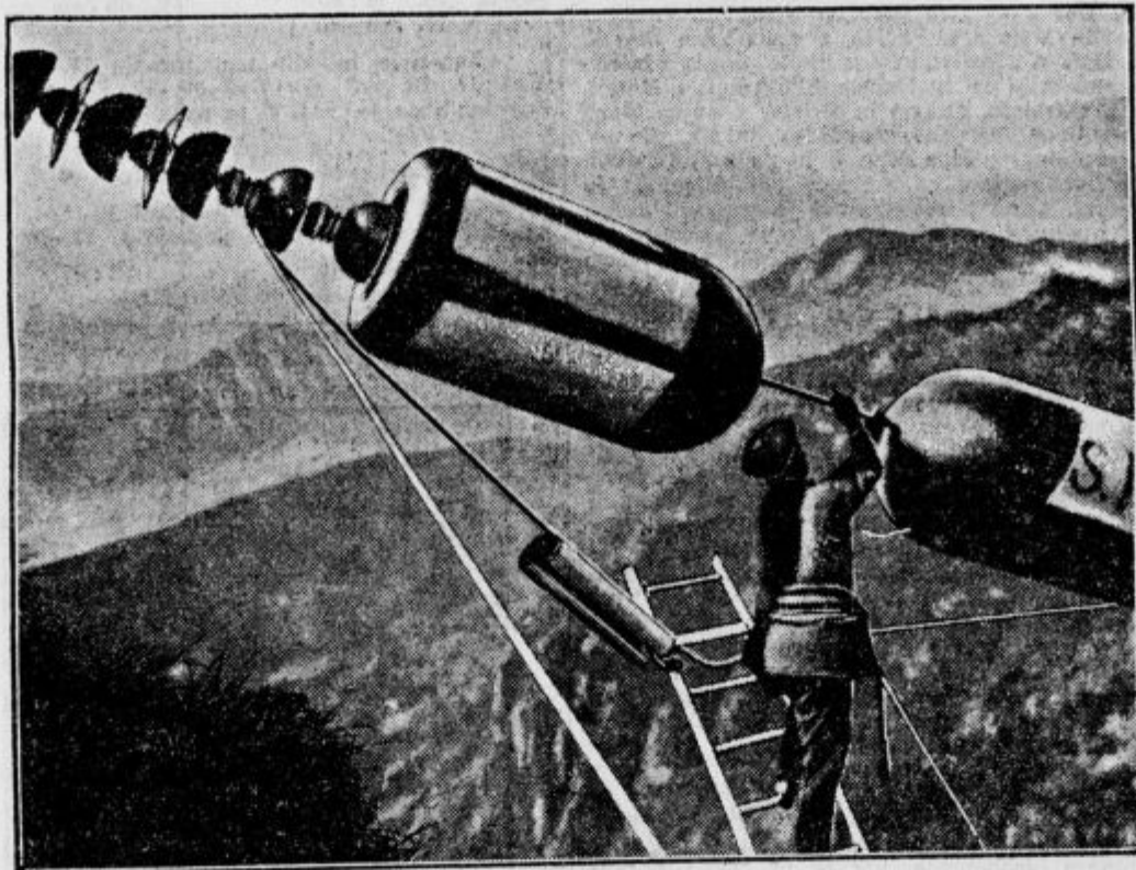
Montaža verige izolatorjev in strelolovcev na Monte Generoso. Berlinski fizikalni inštitut hoče s to napravo zajeti orjaške naravne vire električne sile in z njimi rešiti vprašanje o razbitju atomov.
