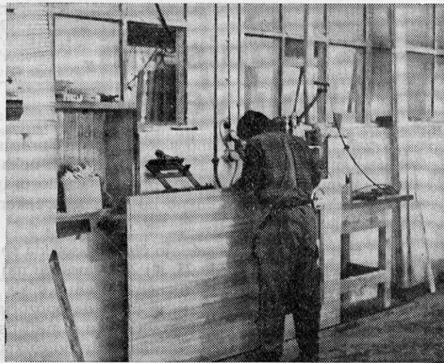
Vrtanje za ključavnico in montaža nasadil se opravlja pretežno ročno
