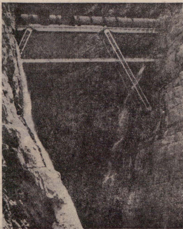
MOST , ki velja za najdržnejše delo italijanskih tehnikov. Pod njim je tristo metrov globok prepad, pri graditvi pa so morali pomagati najbolj izkušeni italijanski alpinisti. Most stoji pri Vaiontu, tam, kjer je prišlo lani do katastrofalnega izlita jez.
