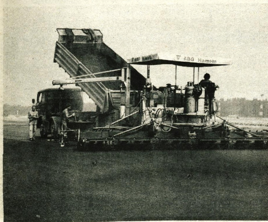
Orjaški finišeji so na brniškem letališču dnevno vgradili na vzlet-nopristajalno stezo nad 4000 ton asfalta — Foto: F. Perdan
