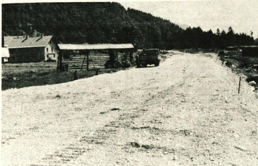
RATECE — Delavci Cestnega podjetja Kranj gradijo novo cesto od Podkorena do mejnega prehoda v Ratečah — Foto: F. Perdan
