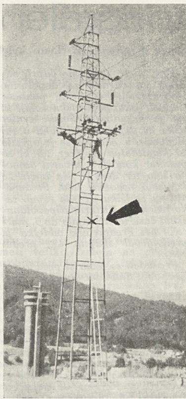
Puščica kaže mesto, kjer je bil kabelski priključek prebit
