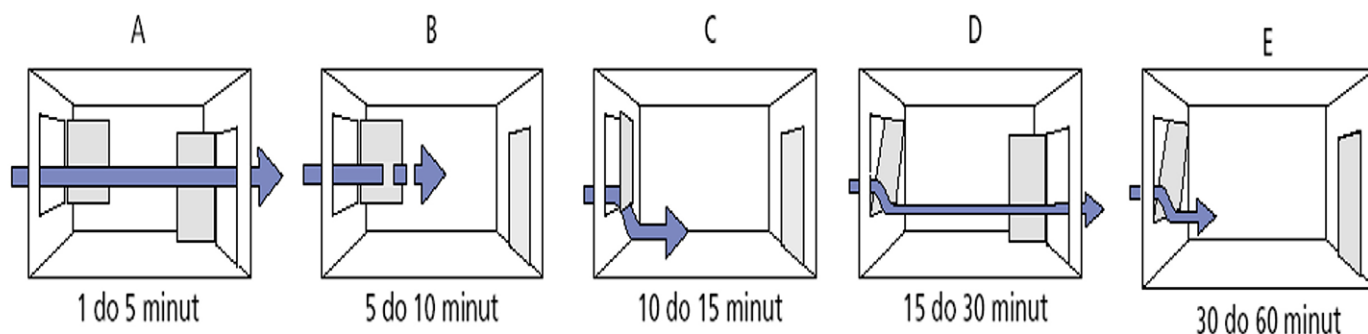
Učinkovitost različnih načinov prezračevanja
