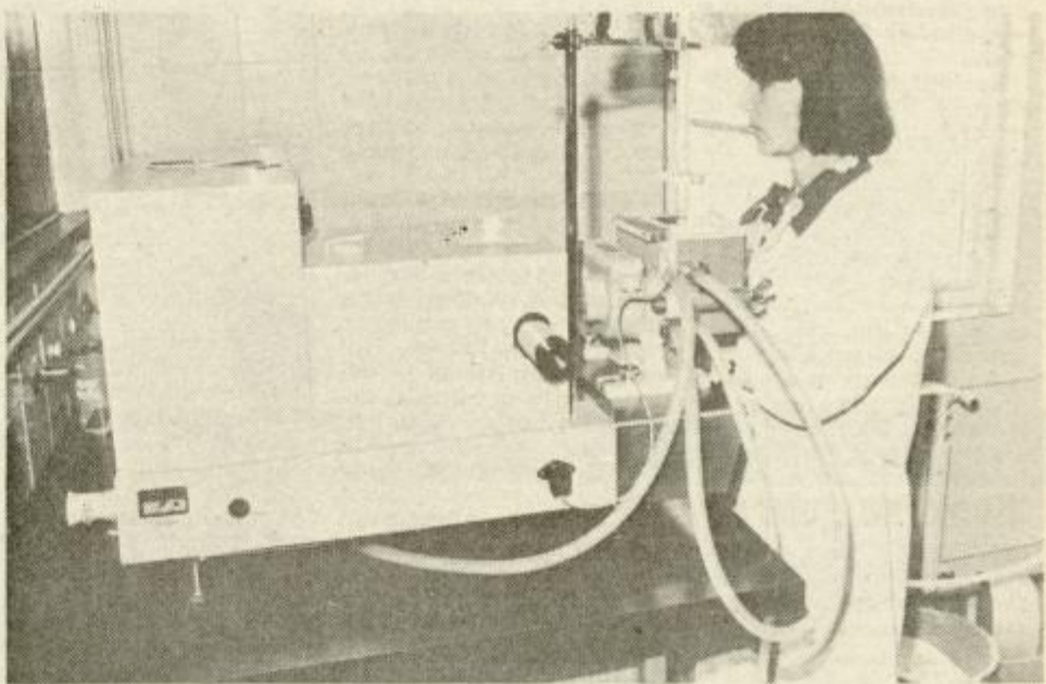
Parinograf, povezan z računalnikom, daje krivuljo kvalitete moke.
