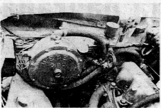
REGULATOR — Namestitev uplinjevalnega-reducirne regulatorja v motornem prostoru. Zraven je elektromagnetski ventil s filtrom za butan in dotočno cevjo; vidimo tudi cevno povezavo regulatorja z ogrevalno vodo iz glave motorja. Foto: EDI SELHAUS
