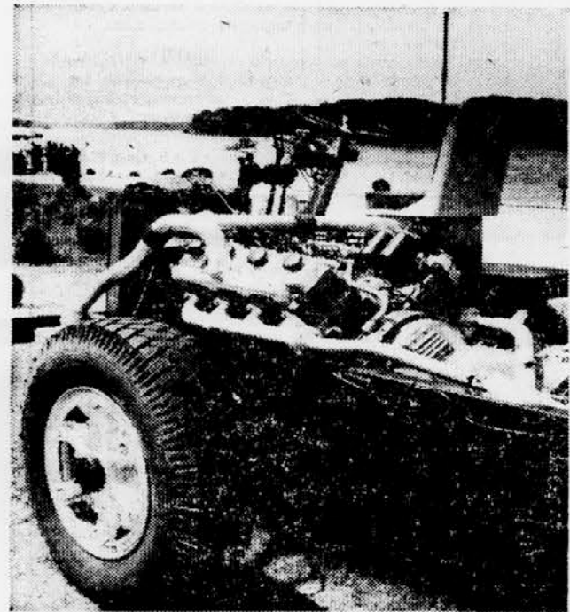
MOTOR »TORPEDO« T-528, 200 KS, 2000 o/min., vgrajen v šasijsko »OM« ORIONE in SUPER, ALFA ROMEO in MILLE. Lastna izdelava motorjev, brez licence.
