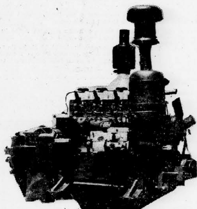
DIESEL MOTOR »TORPEDO« 524 VJ ZA TRAKTOR GOSNICA DT-54 in BNT-60, 705 KS, 1850 o/min.
