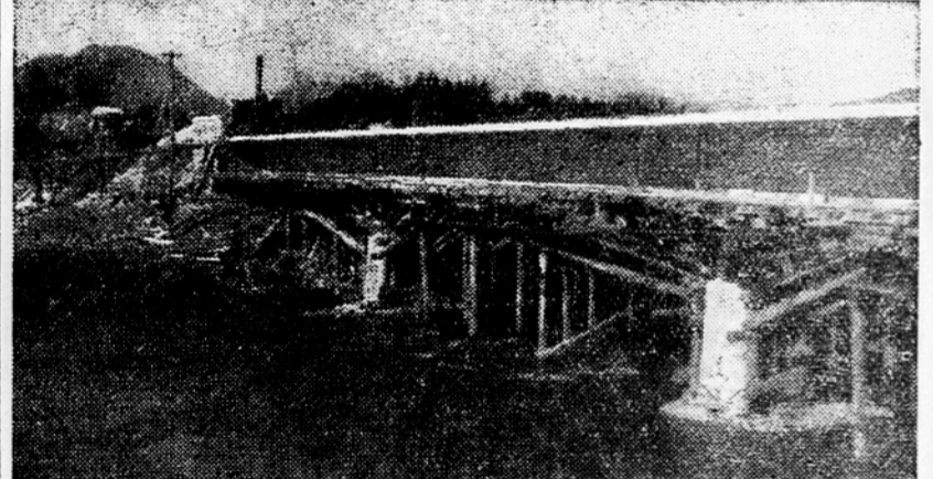
Te dni je bil dokončno obnovljen in izročen prometu cestni most čez Savinjo pri Orli vasi v Savinjski dolini. Obnovljeni most je velikega pomena za razvoj prometa na naši najvažnejši cesti Ljubljana-Maribor.
