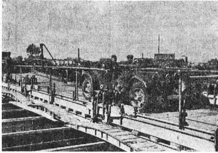
Prehod težkih motoriziranih edinic čez zasilni most
