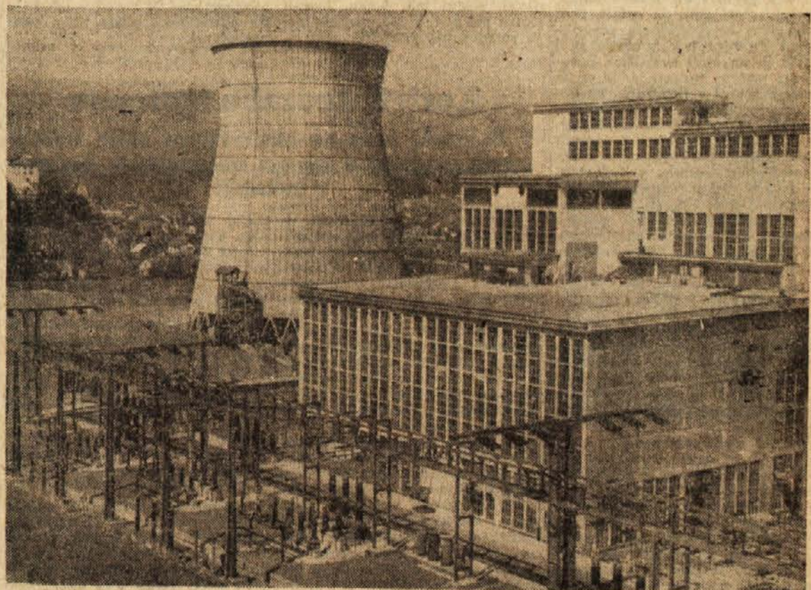
Pogled na del nove termoelektrarne v Sošanju, kjer bodo v prihodnjih dneh zakurili prvi kotel. V obratni stavbi na desni, ki sega do 43 m v višino, sta pripravljena za obratovanje prvi kotel in prvi agregat. Stožčasta betonska stavba na levi je orjaški hladilnik, ki s svojimi 62 metri dosega višino Ljubljanskega gradu, spodaj pa vidimo del razdelilne in transformatorske naprave. (Glej članek na 4. strani)
