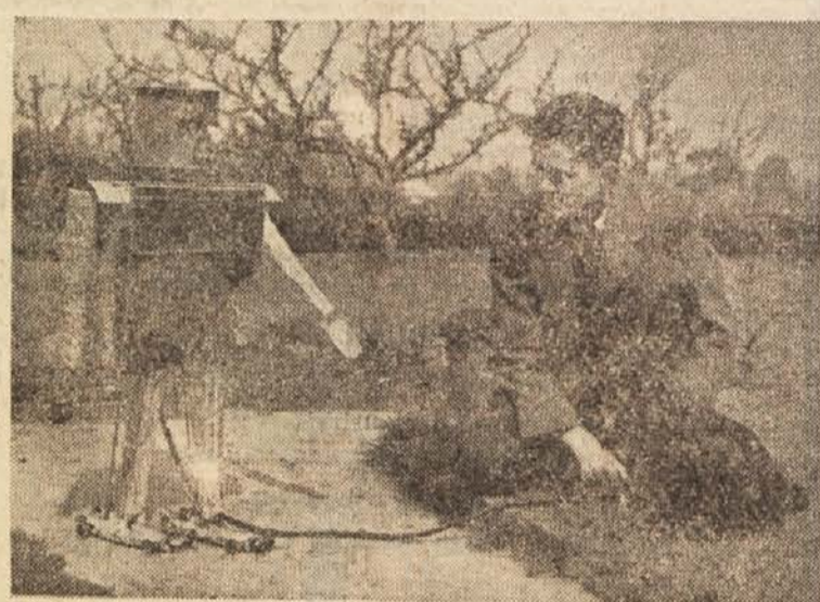
Mladi 17-letni Anglež Frank Grimes, po poklicu tiskar, je izdelal iz starih pločevinastih škatel in stanjov papirja robota, ki ga poganja majhen elektromotor. Robot, ki ga vidimo na sliki, »hodi«, premika obe roki, obrača glavo in suče »oči« -dve električni žarnici
