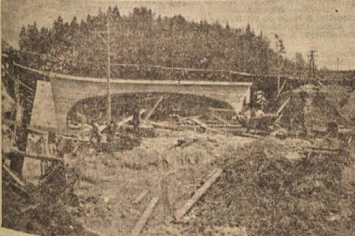
Gradnja železniškega nadvoza nad bodočo avtomobilsko cesto na odseku Skofljica—Šmarje. Objekt grade pod prometom na progih, za frandiranje objekta pa so morali zgraditi pet vodnjakov.
