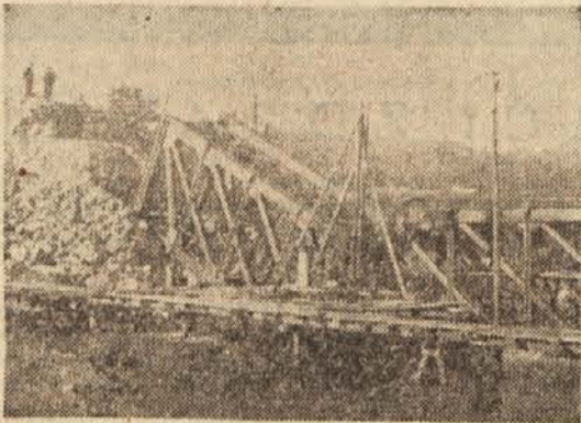
Takšne mostove je pustil okupator
