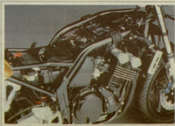
V dvojen cevni Fe okvir nameščeno srce fazerja je izposojeno iz športnika thundercat. Moderen šestnajstventilec s stenami valjev iz keramičnih kompozitov zmore 95 konjev.
