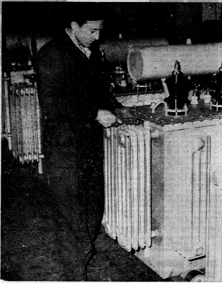
Montaža transformatorja v črnuškem Jamboru
