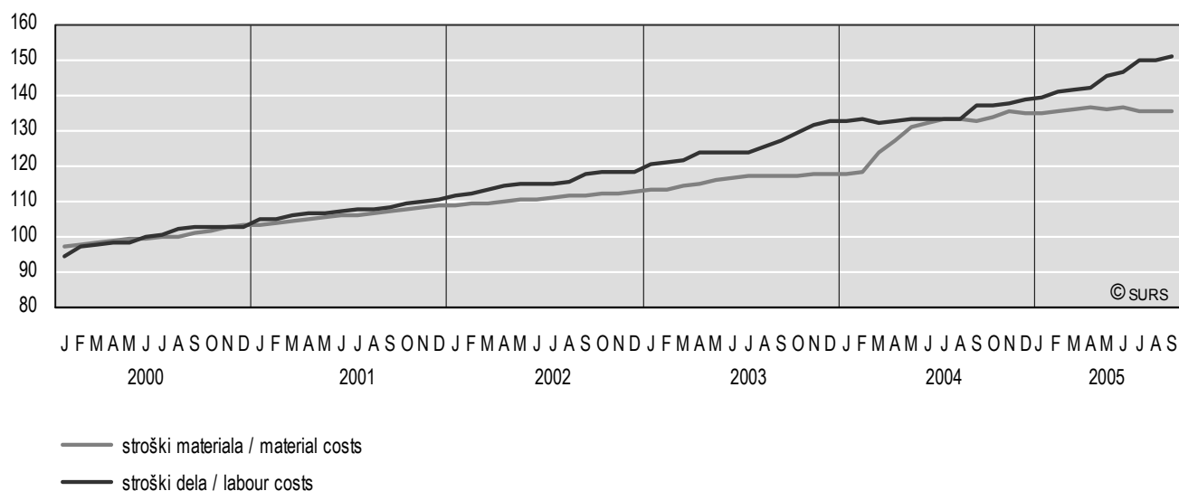
Slika 3: Indeksi gradbenih stroškov, Slovenija, januar 2000 - september 2005
