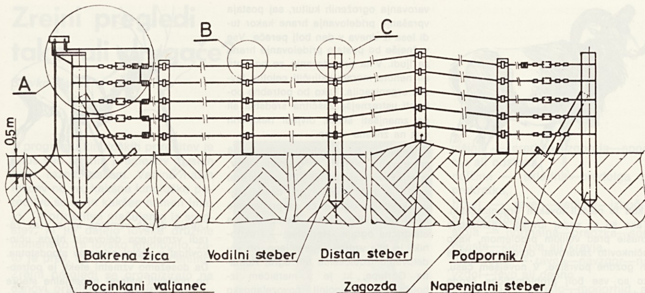
Postavitev učinkovite električne ograje »Herkules — elektronik«
