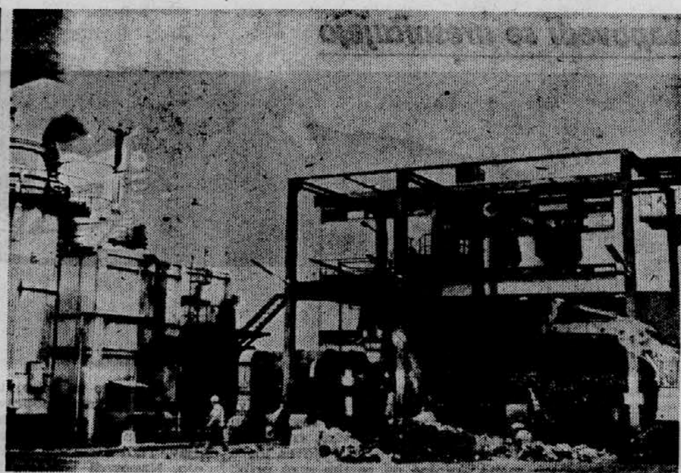
VELIKA PEČ ZA ODPADKE — Strokovnjaki iz raznih dežel si prihajajo ogledovat napravo za sežiganje odpadkov, ki je nedavno začela obratovati južno od Nürnberga. Grajena je v skladu s predpisi o varstvu okolja, v njej sežigajo predvsem nevarne industrijske odpadke, sintetične materiale in kemije snovi, ki jih ni mogoče puščati na smetišču. Celotna naprava je stala pet milijonov mark.
