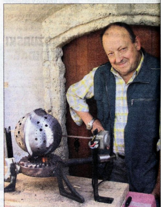
Nevskadnja naprava za peko kostanja. Izdelal jo je Ivan Rošer iz Nove Cerkve.
