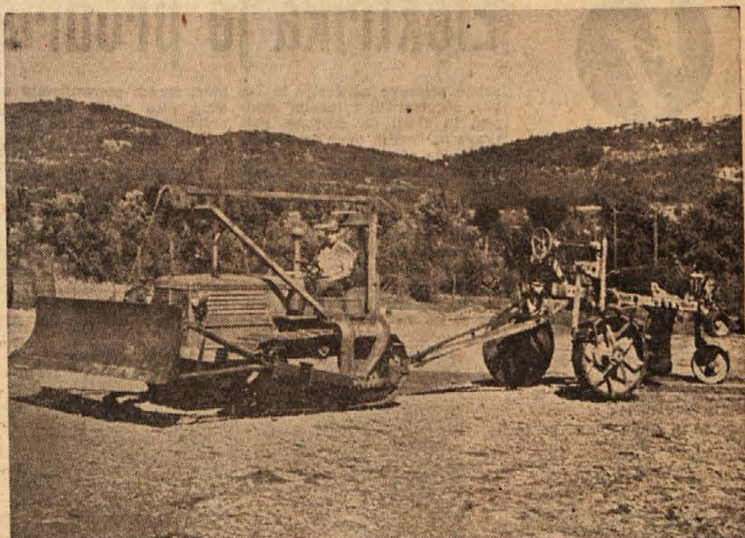
Garnitura za rigolanje vinogradov
