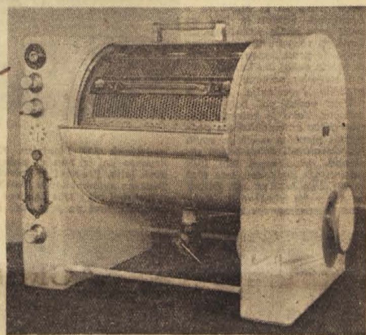
To je pralni stroj z zmogljivostjo 25 kg suhega perila. Doslej so izdelali dva prototipa, ki ju v kratkem dobi Splošna bolnišnica v Mariboru. Ta tip stroja opere 25 kg suhega perila v poldrugi uri. Njegovo poskusno obratovanje je pokazalo, da ga lahko v 8 urah (petkrat) koristno napolnijo. Stroj je dolg 1375 mm, širok 940 mm in visok 1270 mm.
