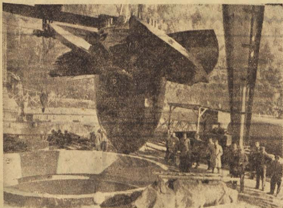
Tako so monterji mariborskega podjetja »Hidromontaže« nedavno tega spuščali v prvi turbinski steber dravske hidroelektrarne Vuhred 50 ton težek tekač Kaplanove turbine.
