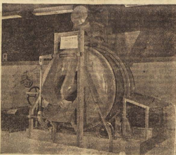
Stabilni betonski mešalec z zmogljivostjo 1000 litrov, je prikladen za večja gradbišča. Izdelujejo ga po potrebi, stane pa 2.800.000 din.
