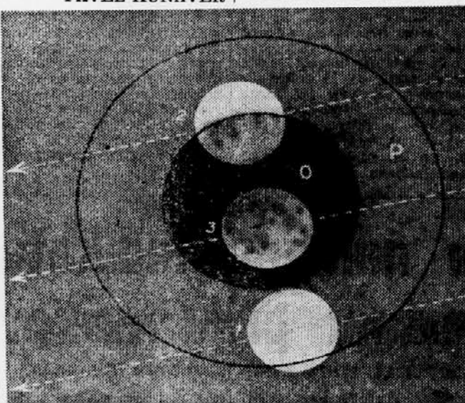
TRI GLAVNE VRSTE Luninih mrkov: O — jedro Zemljine sence; P — polsenca; 1 — posenčni mrk; 2 — delni mrk; 3 — popolni mrk.
