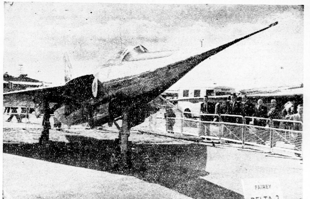
Fairey »Delta 2« — poskusno letalo za nadzvočne hitrosti. Značilna so delta krila, namočena na zadnjem delu trupa in dolg koničast nos, ki je konstruiran tako, da se pred vzletom dvigne, pri pristajanju pa povesi in omogoči pilotu pregled nad vzletno stezo. Letalo poganja reaktivski motor »Avon« tvrdke Rolls Royce, ki razvije potisno silo, da letalo v vodoravnem letu prebije zvočni zid.
