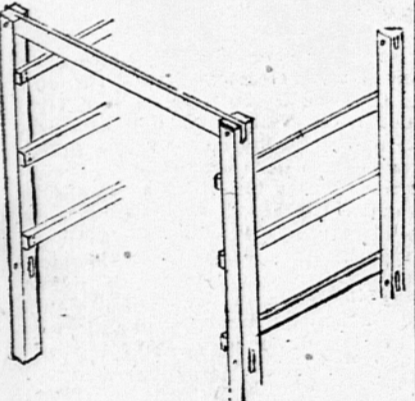
Sušilno ogrodje, sestavljeno iz dveh stolov, od katerih ima vsaka po tri prečke za lese. Stojali sta povezani z odstranljivimi vetvami.
