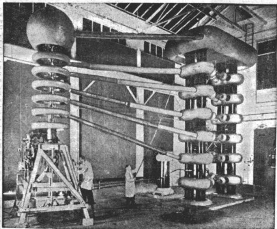
NAJVEČJI RÖNTGENSKI APARAT. V Moabitu pri Berlinu so montirali največji röntgenski aparat na svetu. Naprava, ki zdrži napetost 1.200.000 voltov, je namenjena za zdravljenje raka. Žarilna moč aparata odgovarja sili 10 kg radija
