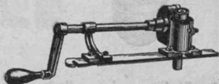
Št. 166. Gonilo za točilo, najnovejšega sestava za pogon s strani:
