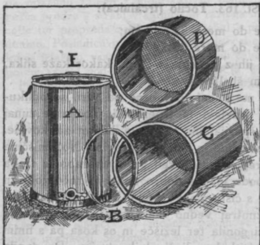
Št. 170. Čistilnik za med za večji obrat.
