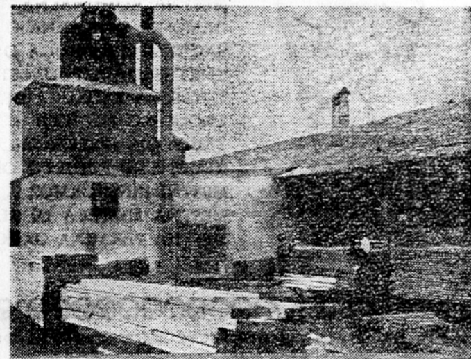
Izbira desk pred sušilnico s silosom za žagovino in lesene ostružke
