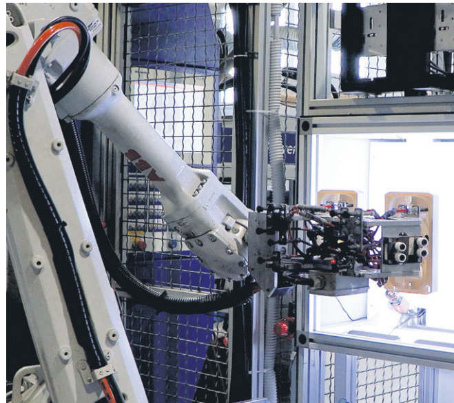
Šest kamer za 360-stopinjski pregled izdelkov in programa za prepoznavanje kakovosti. (Foto: Skaza)
