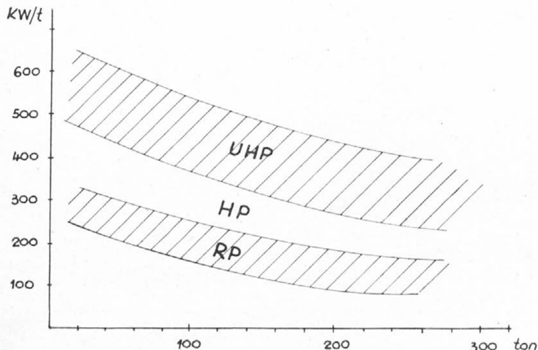
Sl. 1 Območja specifične moči obločnih peči
