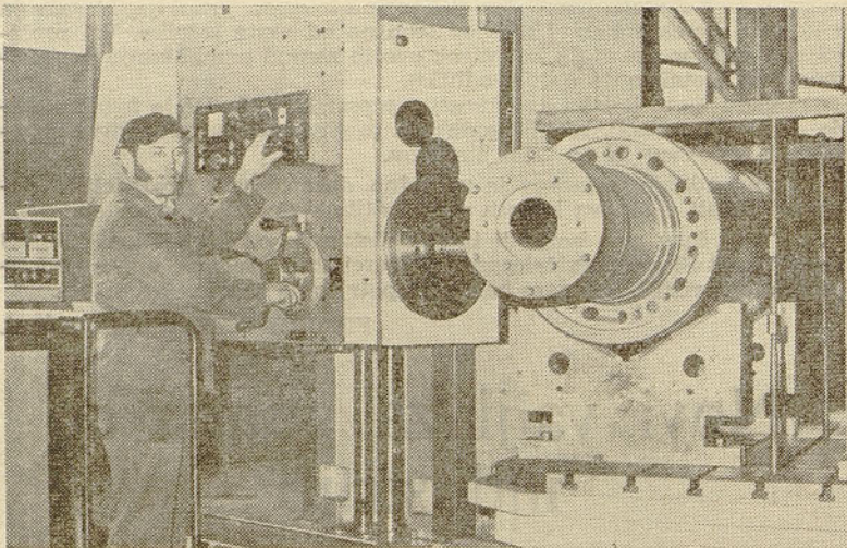
Zaključna faza obdelave — vrtanja kanalov na valju za potrebe gumarske industrije, nov dosežek naših strokovnjakov
