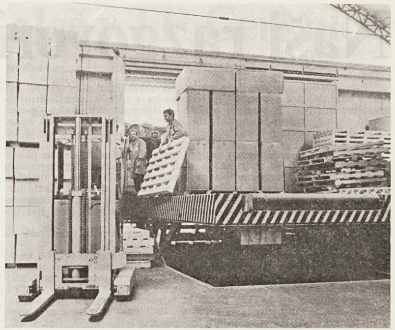
Nakladišče v novih skladiščnih prostorih
