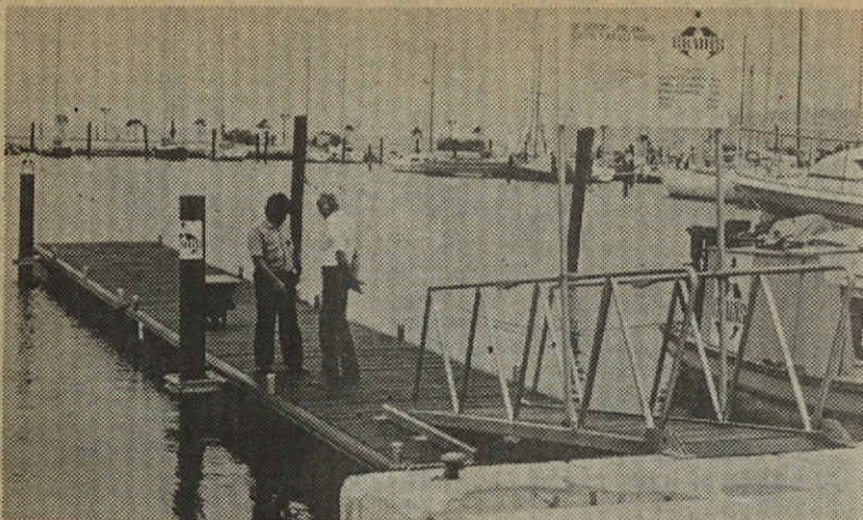
Prototip plavajočega pomola širine 2,5 m v marini Portorož
