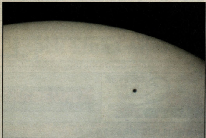
Slika Merkurja na Soncu
