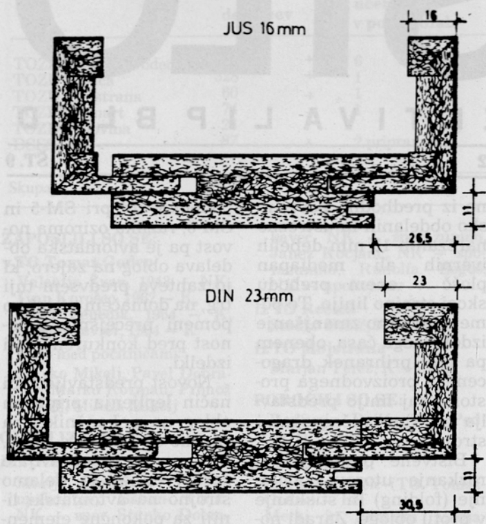
Profil novega podboja uspešno rešuje prilagajanje različnim odstopanjem v debelinah zidu
