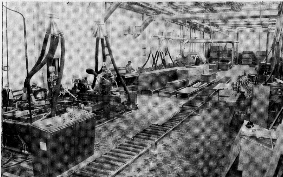
Poskusna proizvodnja oblog po sistemu folding
