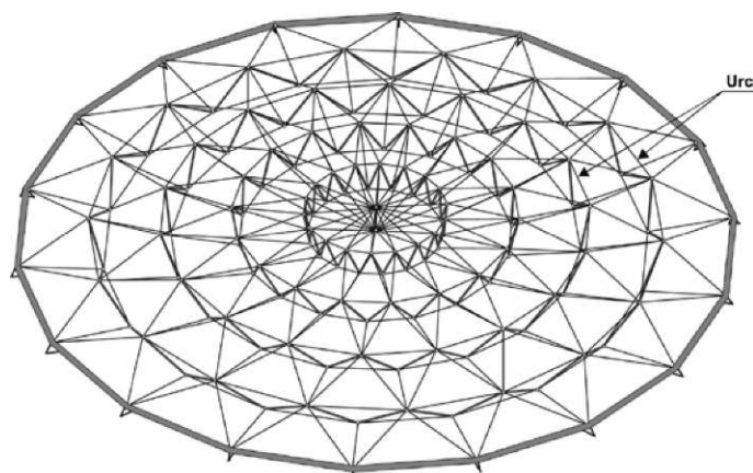
Slika 3: Splošni pogled na osnovno obliko konstrukcije nateznikov. Figure 3: General view of the basic form of the crystal tension-strut structure.
