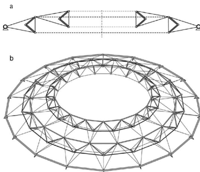
Slika 5: Primer oblike konstrukcije nateznikov tipa VU-TensO. a) shema glavnega vertikalnega prereza, b) pogled na celotno konstrukcijo kupole. Figure 5: Example shape of the tension-strut structure VU-TensO. a) scheme of the main vertical cross-section, b) overall view of the dome structure.
