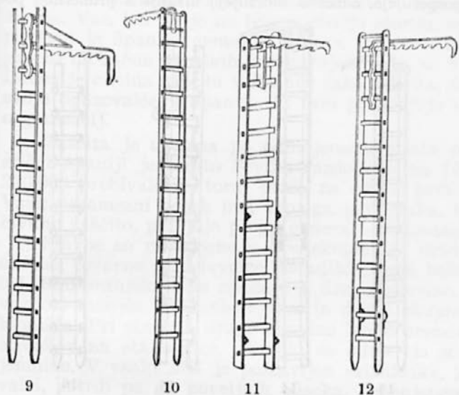
9.—12. Kljukaste lestve z žagasto kljuko v raznih izvedbah
