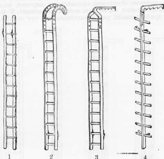
1. Navadna lestev — 2. Kljukasta lestev s krožno kljuko — 3. Kljukasta lestev z žagasto kljuko — 4. Kljukasta lestev z enim lestvenikom
