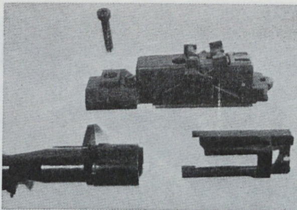
Ohišje zaklepa, premični mostiček, vodilo z magazinom, mehanizmom za proženje in ležiščem glave; glava je povezana s cevjo
