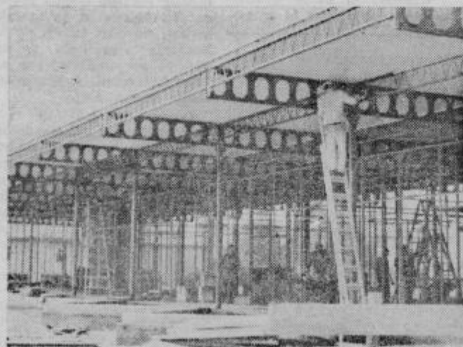
Gradbeno podjetje »Drava« končuje dela pri gradnji nove avtobusne postaje.
