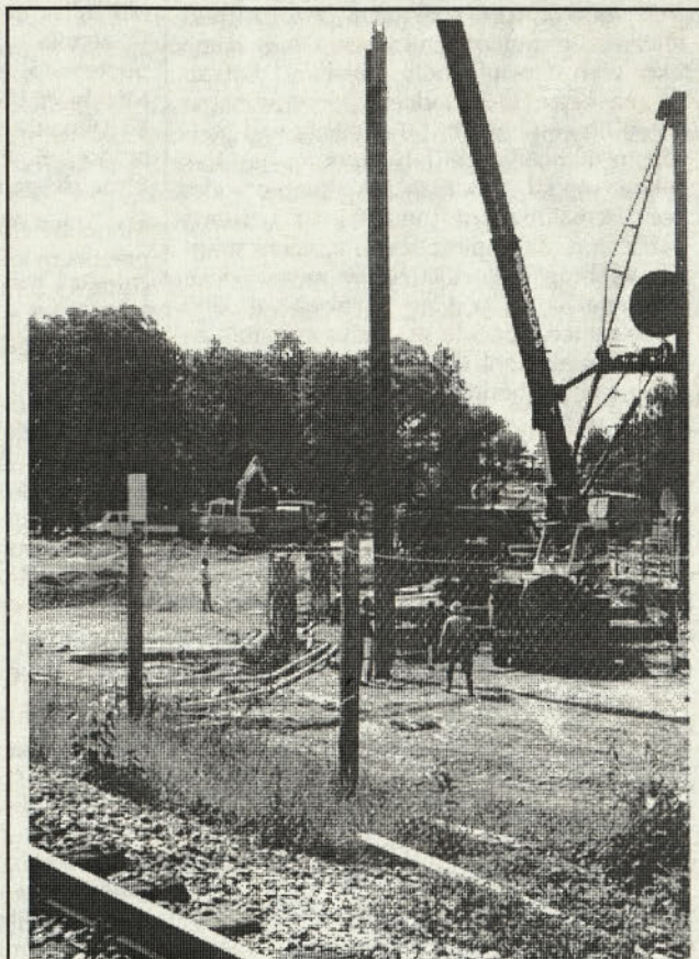
Kopanje jame za podvoz v smeri mostu.
