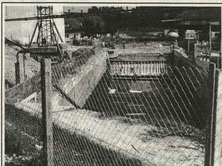
Gradbena jama od železnice proti Ormoški. Vidni sta membranski steni in črpanje podtalnice po sistemu natege.
