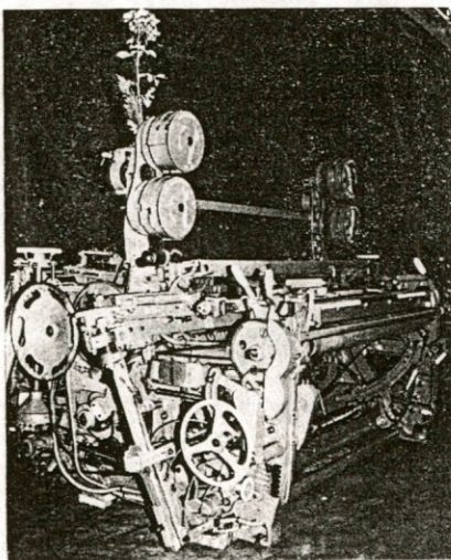
Obnovljen tkalski stroj
