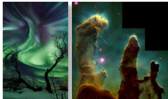
Živahen severni sij nad Norveško
