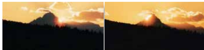
Vsako leto si iz našega observatorija 20. ali 21. junija ogledamo znameniti »dvakratni« sončni zahod za Triglavom.
