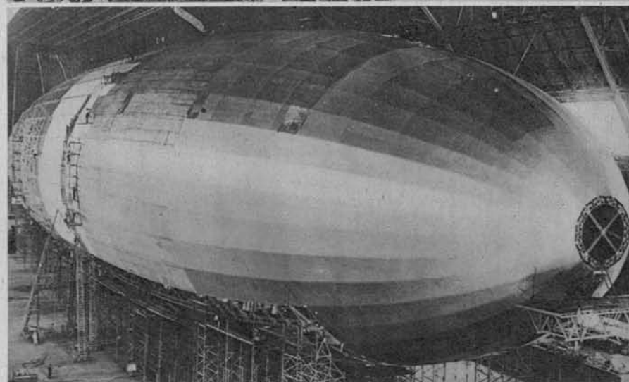
Največji zrakoplov sveta grade sedaj Američani in bo v nekaj tednih dovršen. Dolg bo 785 čevljev (torej še enkrat večji kot »Zeppelin«), nosil bo lahko 91 ton tovora, njegova hitrost bo znašala 135 km na uro, letel bo pa lahko 18.000 km brez prestanka. Njegovo ogromno razsežnost spoznamo lahko iz primerjave med avtomobili na tleh in zrakoplovom.
