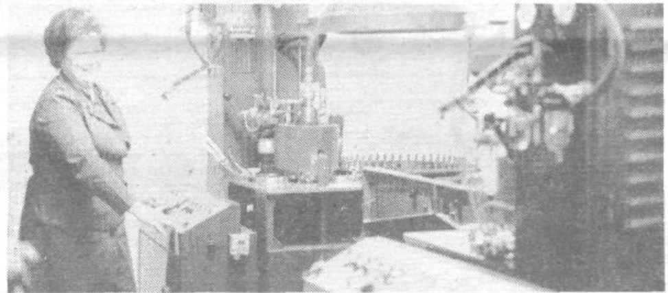
Nad 40 milijonov vredna popolnoma sinhronizirana linija SACMI za izdelavo navojnih zapork 28 krat 15 mm bo nekaj mesecev kovala te zelo iskane zaporke v začasnih prostorih stare delavnice za izdelavo aluminijastih zapork. Pričakujejo, da bo lahko stekla na stalnem mestu v veliki proizvodni dvorani proti koncu letošnjega leta.
