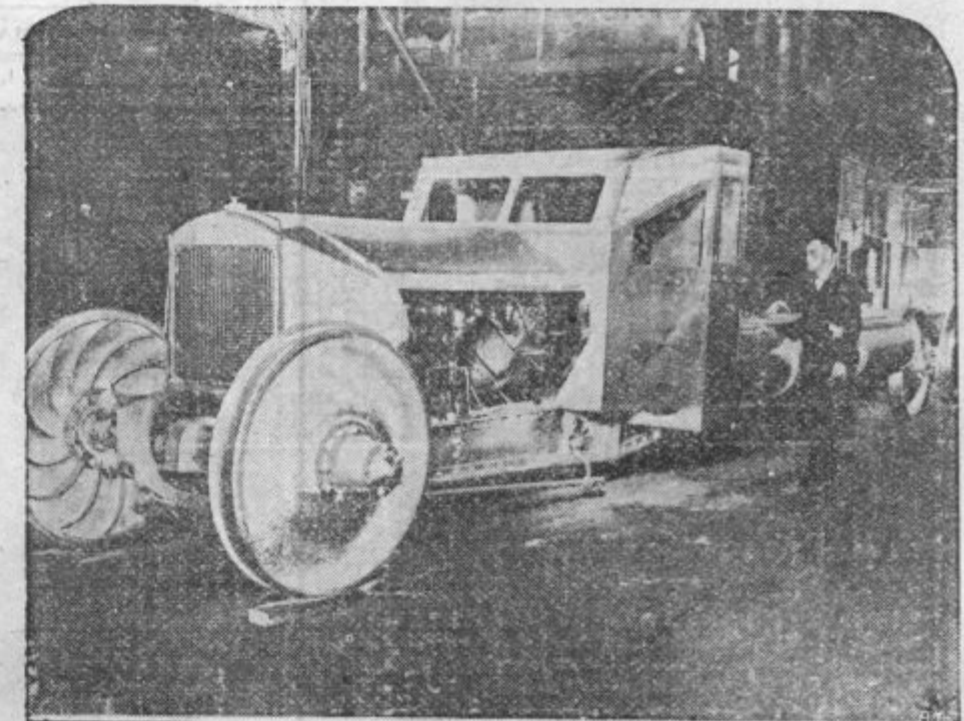
AVTO BREZ KURIVA. V Atlanti (USA) so skonstruirali motorno lokomotivo, ki ovozila s povprečno brzino 200 km na uro. Najzanimivejše pri novem vozilu je to, da ga ne poganja nobeno kurivo, temveč stisnjeni zrak. Stroški za napolnitev baterije, ki proizvaža potrebni stisnjeni zrak, znašajo komaj 2,48 dolarja.
