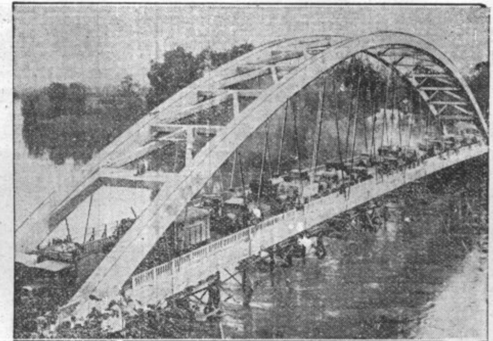
NAJVEČJI MOSTNI LOK NA SVETU. V Franciji so izročili prometu most v Castel-moronu. Most ima samo en lok in meri v dolžino 140,40 m ter je največji na svetu.
