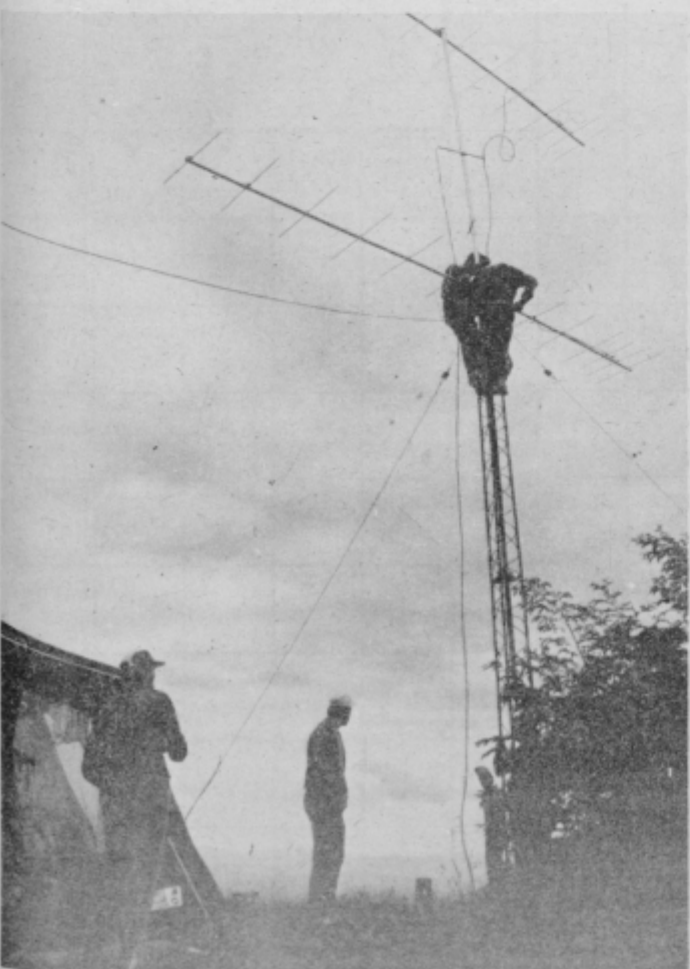
Montaža anten na stolpu na vrhu Donačke gore
