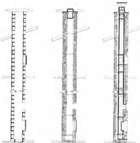
skica 4: možne izvedbe suhega dimnika
