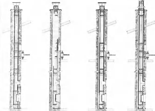
skica 5: možne izvedbe vlažnega dimnika
