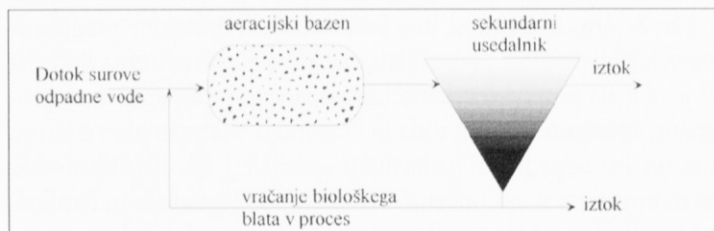
Postopek čiščenja odpadne vode z aktivnim blatom
