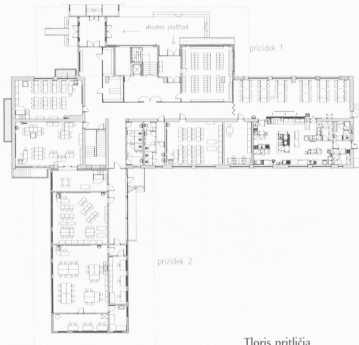
Tloris pritličja
