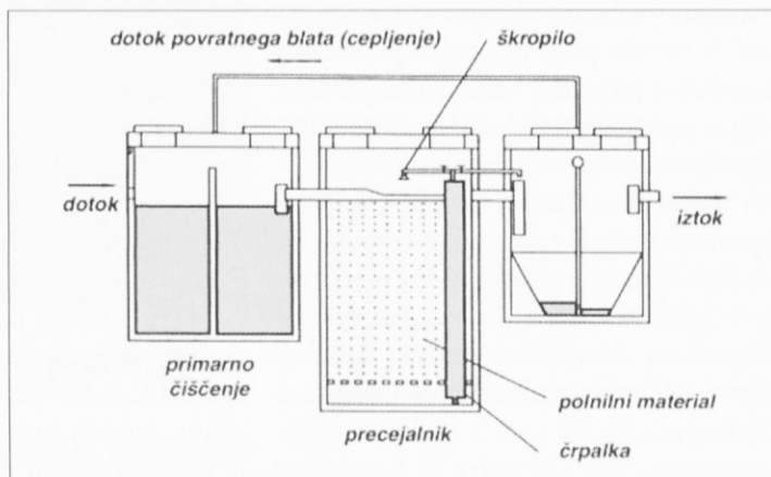
Mala čistilna naprava s precejalnikom
