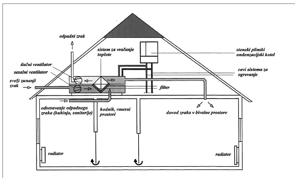
Shema sistema ogrevanja, priprave sanitarne vode in prezračevanja z vračanjem toplote (rekuperacija toplote)
