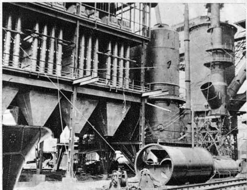
Pogled na moderni plavž. Debele cevi služijo za odvajanje izgorelih plinov, da se morejo nadalje izrabljati.
