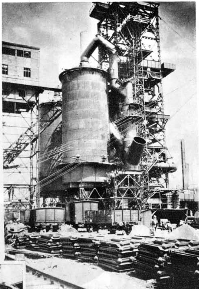
Pogled na moderni plavž. Debele cevi služijo za odvajanje izgorelih plinov, da se morejo nadalje izrabljati.
